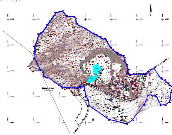
Figura nº 8: Levantamento topográfico
