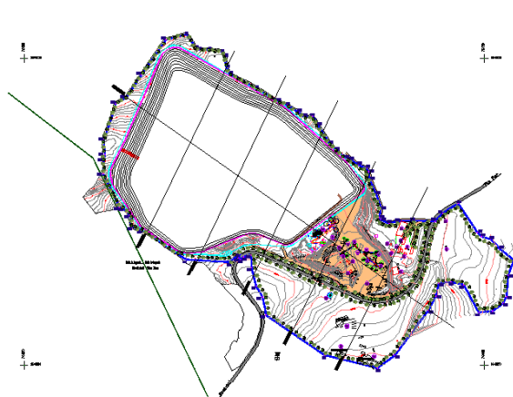
Figura nº 10: Situação final de exploração
